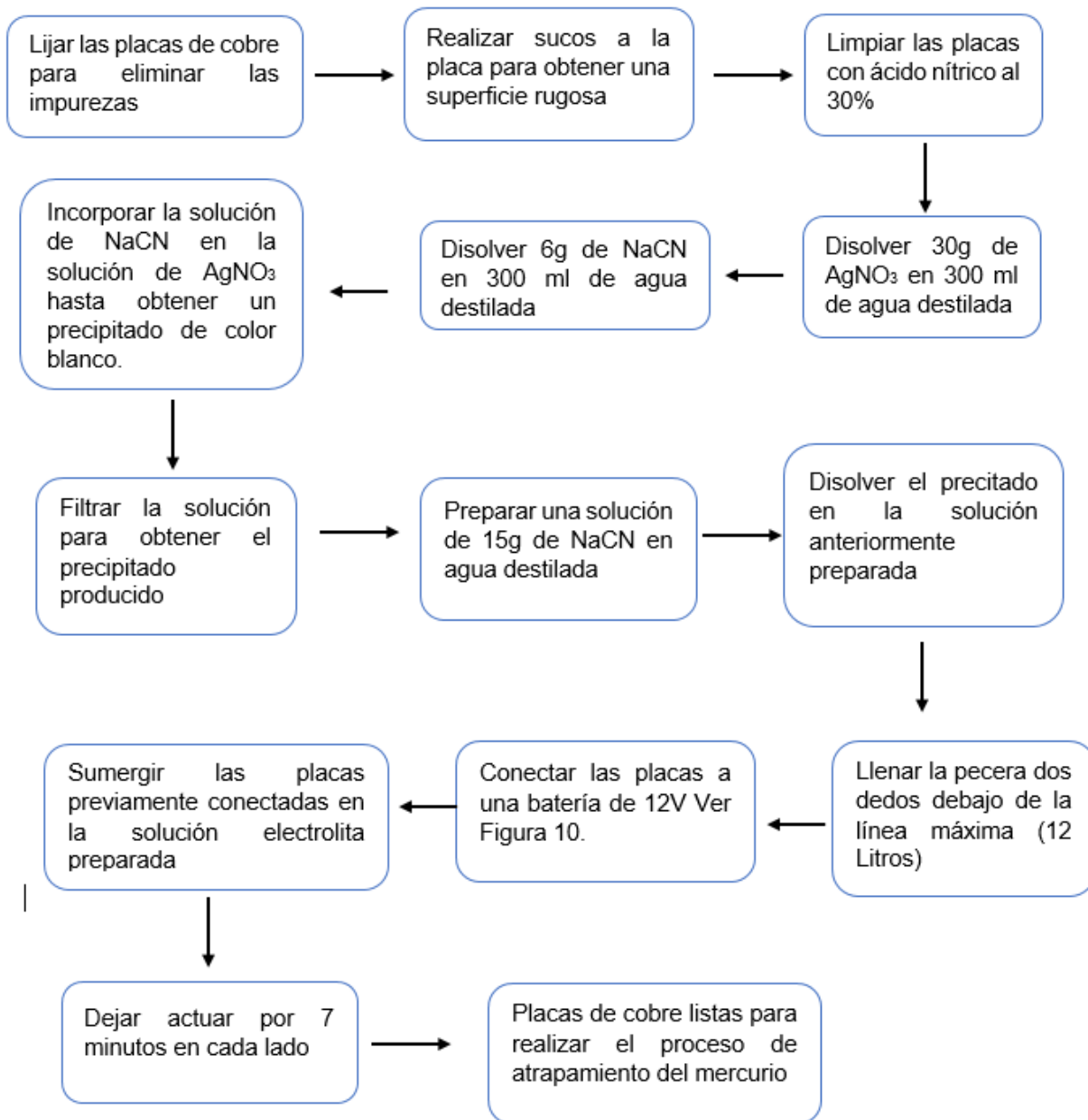
Figura 9. Procedimiento para la fabricación de las placas de cobre amalgamadas con plata
