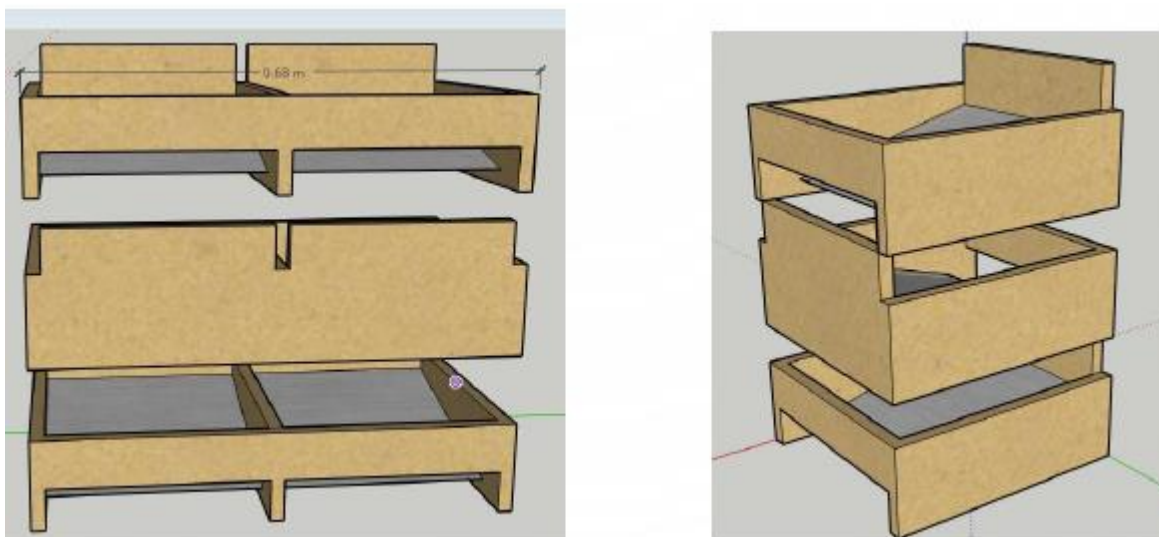
Figura 18. Prototipo módulo de soporte de las placas de cobre
