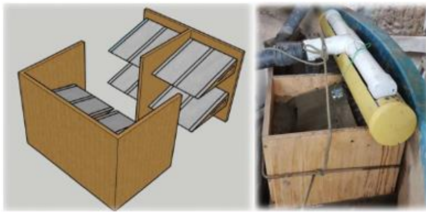
Figura 13. Módulo de soporte de las placas de cobre y circuito de distribución de flujo
